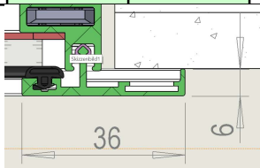
Abdeckrahmen flach
