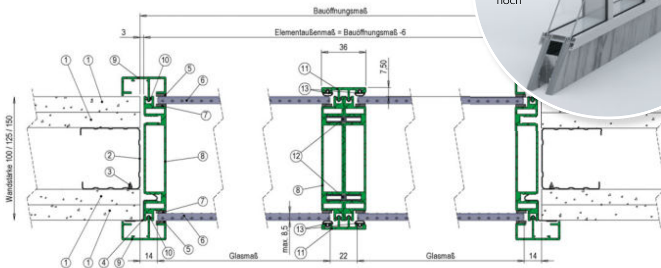
Verkettungs- element Rahmen hoch
