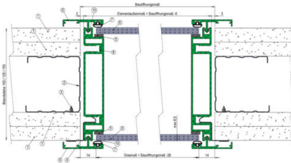
Einzelement Rahmen flach
