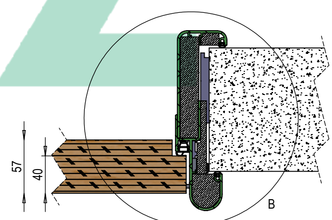
SCHNITT A-A MAßSTAB 1 : 4
